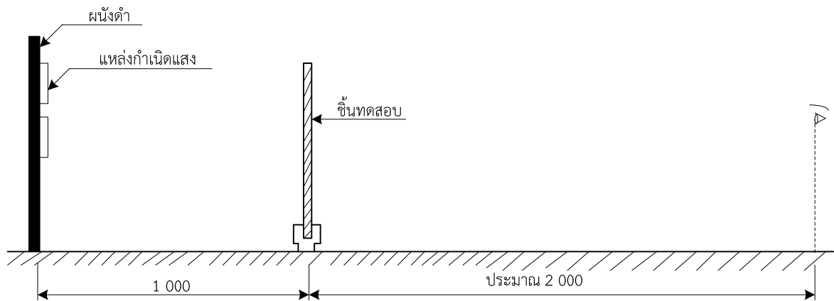
รูปที่ 1 การทดสอบรายการฟองอากาศ สิ่งแปลกปลอม ดำหนดเป็นจุดรวมเป็นกลุ่ม ดำหนดเป็นเส้นหรือเป็นปื้น ต่อเนื่องกัน ดำหนดเป็นแนวยาวในเนื้อกระจก ราน สีผิดปกติ และขูดขีด (ข้อ 9.2.2)
