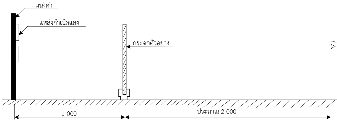
รูปที่ 2 การทดสอบหาค่าหยาบ (ข้อ 9.2.2)
