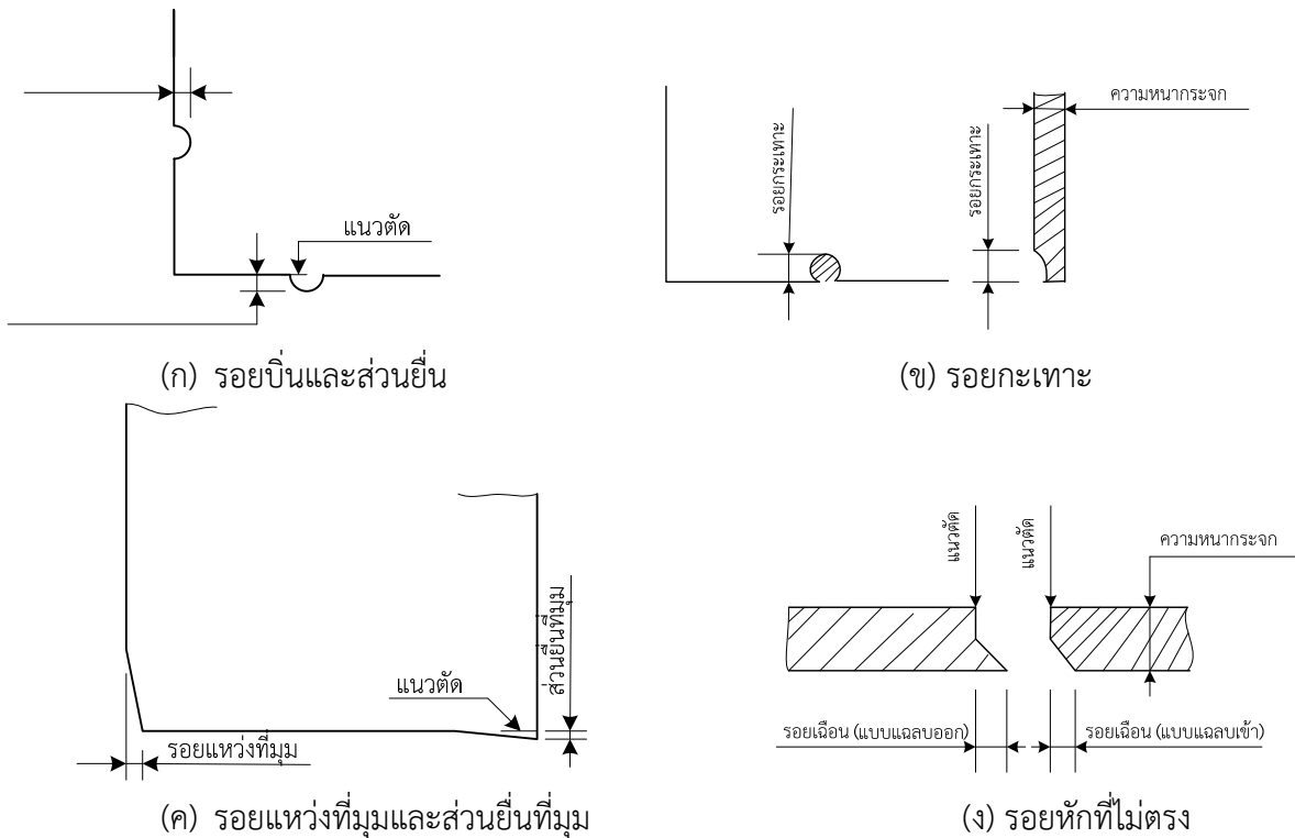
รูปที่ 3 ค่าหยาบที่ขอบ (ข้อ 9.3.2)
