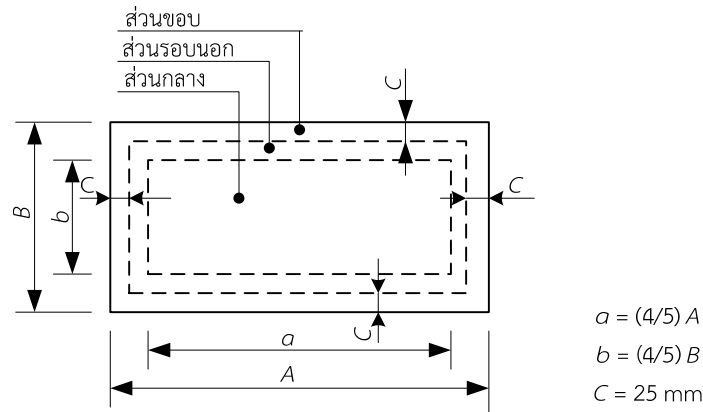
รูปที่ 1 การแบ่งส่วนกลาง ส่วนรอบนอก และส่วนขอบของกระจกโพลีคาร์บอเนตแสง ชั้นคุณภาพพิเศษ (ข้อ 9.2)
